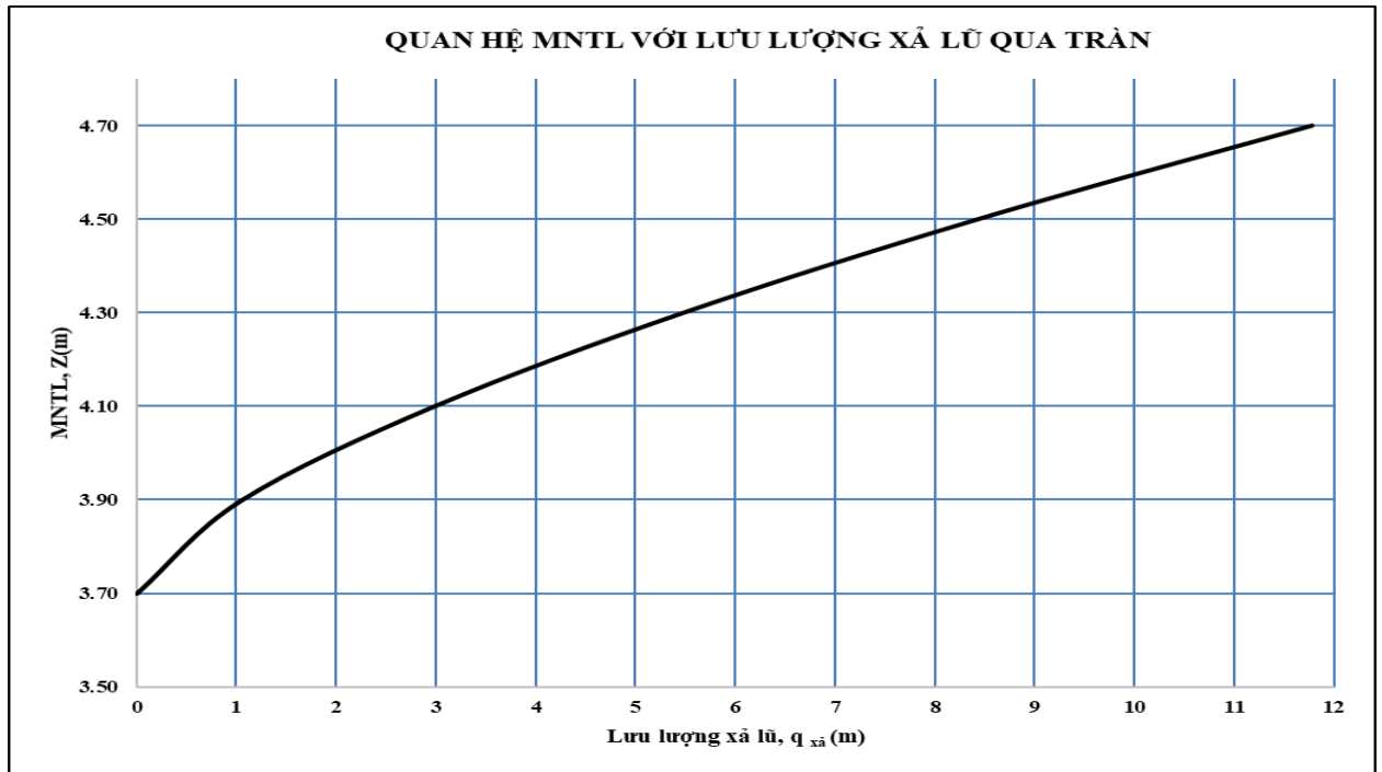
Hình 1: Biểu đồ quan hệ ( Q_{\text{xả}} \sim Z_{\text{hồ}} ) của tràn xả lũ
