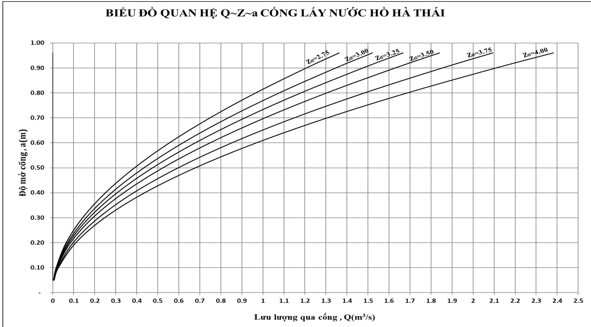
Hình 4: Biểu đồ quan hệ ( Q \sim a \sim Z ) công lấy nước hồ Hà Thái
